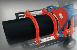
Alin Kaynak Makinası AL 315 CNC
